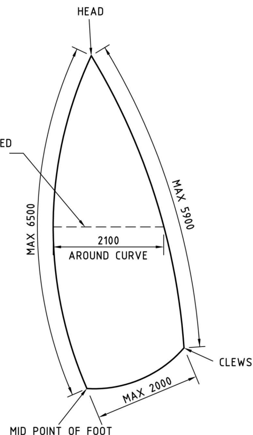
SPINNAKER
