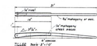
TILLER Scale: 3"=1'-0"
