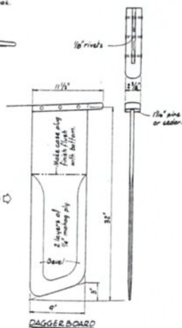
DAGGERBOARD
