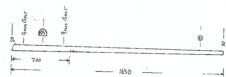
MIZZEN BOOM
